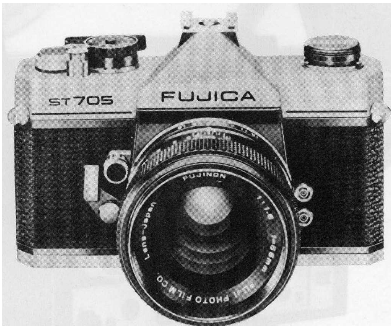
Fujica ST 705 - Reflex 24 x 36 semi-automatique. Mesure à pleine ouverture. Cellule au silicium. Objectifs interchangeables à monture vissante au pas de 42 mm. Prix environ 1 750 F.
