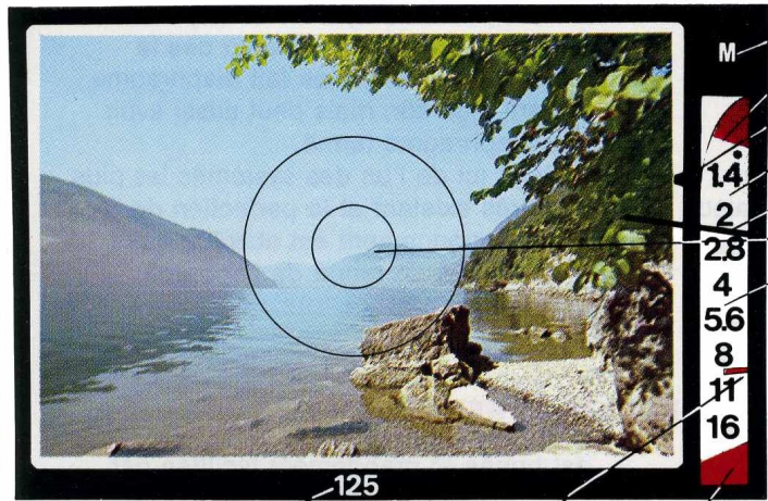
Indication de la vitesse choisie. Repère du contrôle des piles. Zone de sur-exposition.
