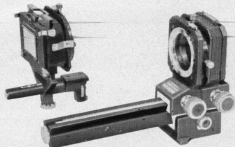
SOUFFLET auto-bellow pour Pentax
