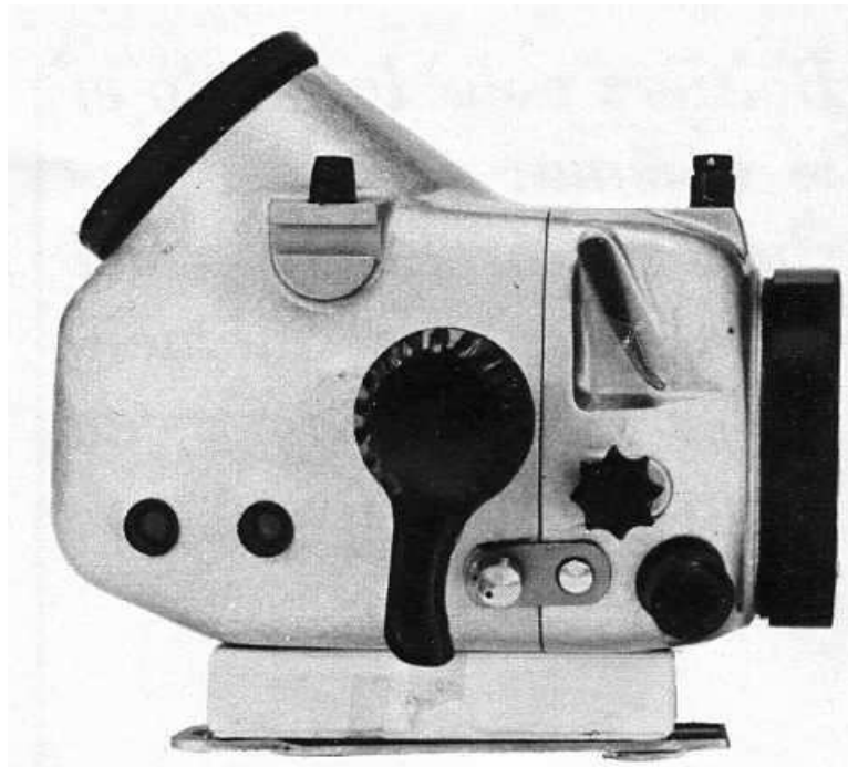
TRITON : boîtier pour Hasselblad exclusivement. Profondeur 120 m. Commandes : toutes. Construit en alliage d'aluminium. Garanti 2 ans. 4 900 F.
