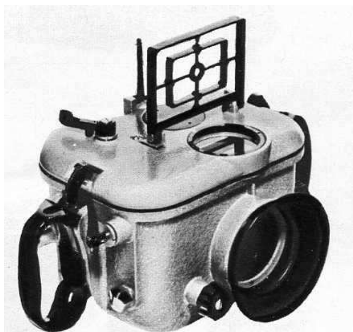
PHOTOSCAF : boîte pour Zénit exclusivement. Profondeur 40 m. Viseur à cadres avec fenêtre reflex. Correction de parallaxe. 800 F.
