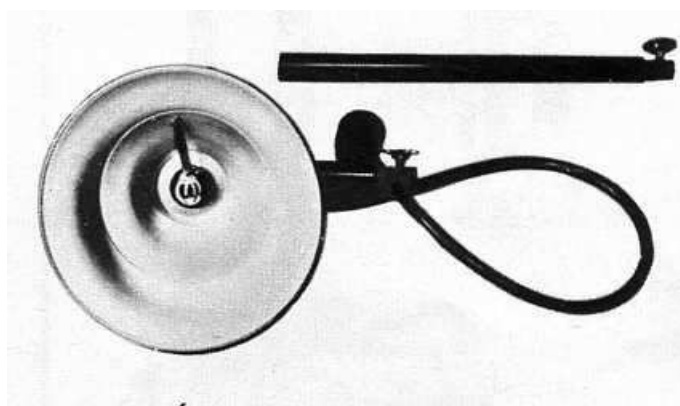
PHOTOCINÉSUB : flash magnésium. Profondeur 50 m. Alimenté par piles blindées. Lampes AG. Réflecteur orientable. 30 F.
