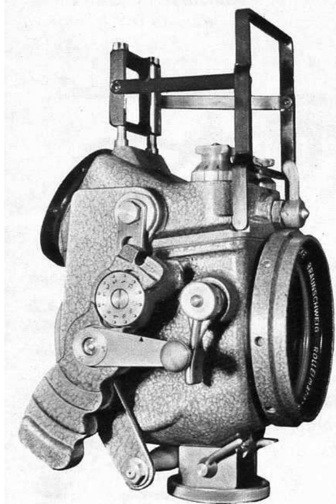
ROLLEI MARIN : boîte étanche pour Rollei. Profondeur 100 m. Commandes : toutes. Préciser le numéro de l'appareil à la commande. 2 400 F.
